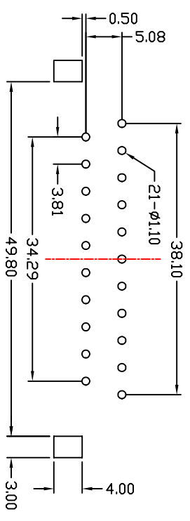
P.C.B. LAYOUT
